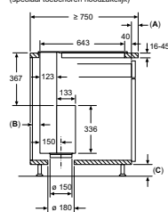
Afmeting in mm Naadloze installatie (speciaal toebehoren noodzakelijk)
