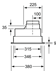
Afmeting in mm
