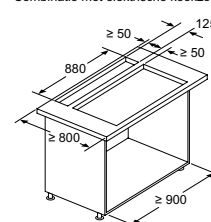
Afmeting in mm Combinatie met elektrische kookzone
