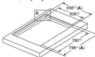
Afmeting in mm Combinatie met elektrische kookzone Naadloze, vlak geïntegreerde inbouw
