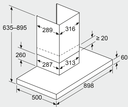
Maße in mm Ansicht Umluft
