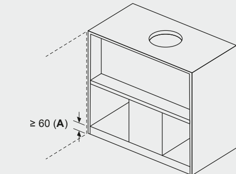
Maße in mm Einbaubeispiel mit Gewürzregal
