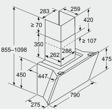
Maße in mm Gerät im Abluftbetrieb
