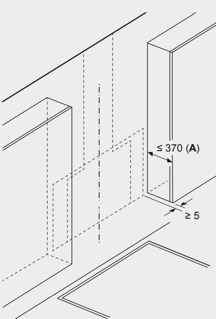
Maße in mm
