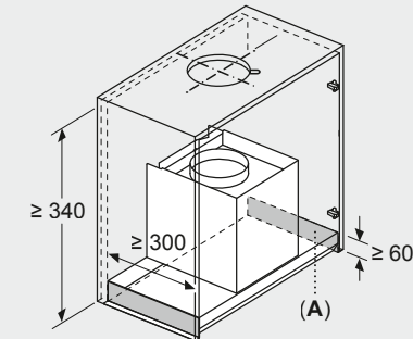
Maße in mm Installationsanforderungen für den Ersatzbedarf
