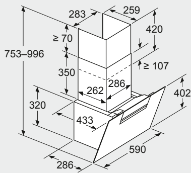
Maße in mm Gerät im Abluftbetrieb
