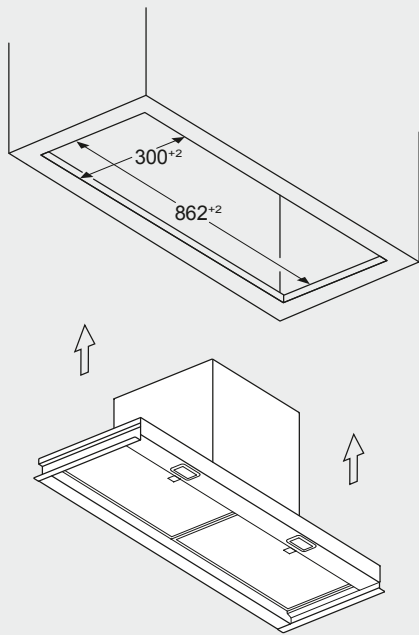
Maße in mm Einbaubeispiel in Möbelausschnitt
