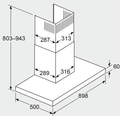
Maße in mm Ansicht Umluft
