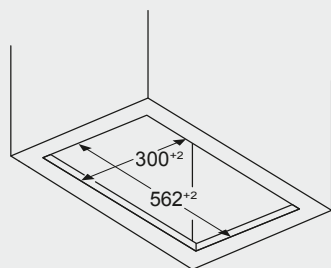
Maße in mm Einbaubeispiel in Möbelausschnitt
