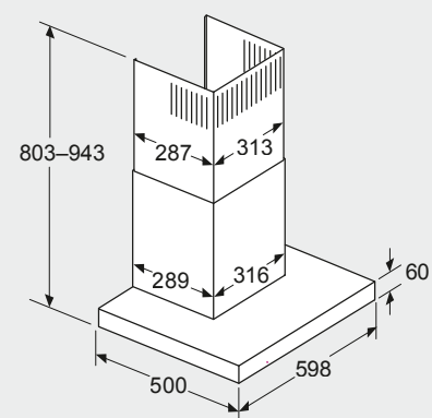
Maße in mm Ansicht Umluft
