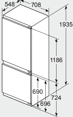
Maße in mm
