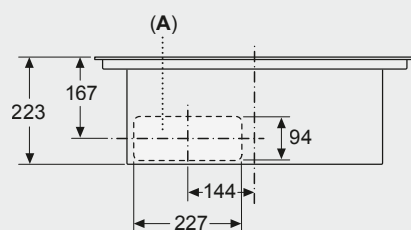
Maße in mm Vorderansicht
