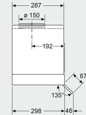
Maße in mm Seitenansicht
