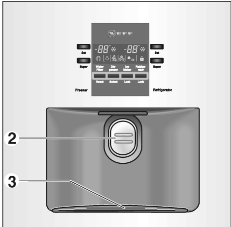
2 Entnahme-Pad 3 Wasser-Auffangschale
