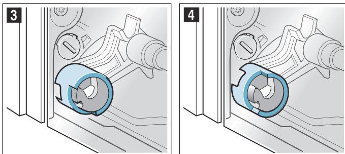
Scharnierverriegelung geschlossen (Bild 3 ) Scharnierverriegelung geöffnet (Bild 4 )
