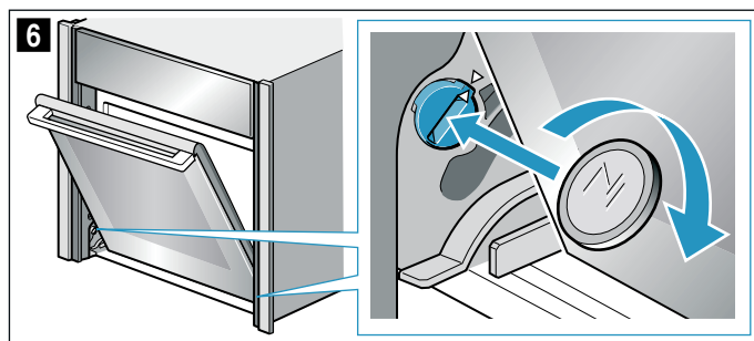
Mecanismul de blocare din partea stângă cuplat (imaginea 7)
