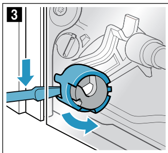
Ασφάλεια πόρτας κλειστή (Εικ. 3 ) Ασφάλεια πόρτας ανοιχτή (Εικ. 4 )
