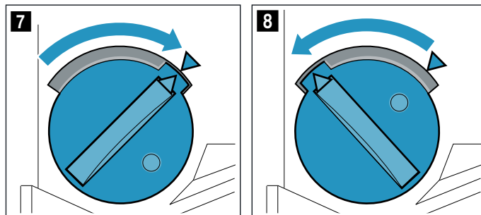
Bal oldali rögzítő kioldva (8. ábra)
