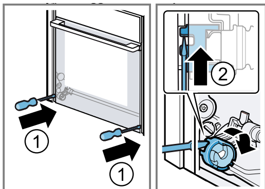
Åbnet dørlåseanordning
