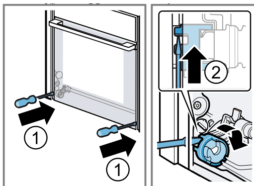
Åbnet dørlåseanordning
