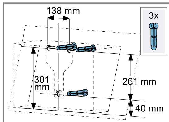
Вариант Б: Скосен абсорбатор без обшивка за димоотвод
