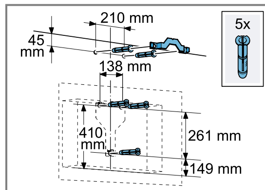
Вариант А: Плосък абсорбатор с обшивка за димоотвод
