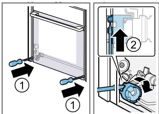
Åbnet dørlåseanordning
