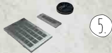
Kit recirculare cu regenerare pentru instalare hotă fără horn Cod: Z51AIR0X0
