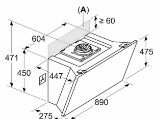
Измерване в mm Уред в режим циркулиращ въздух без димотвод
