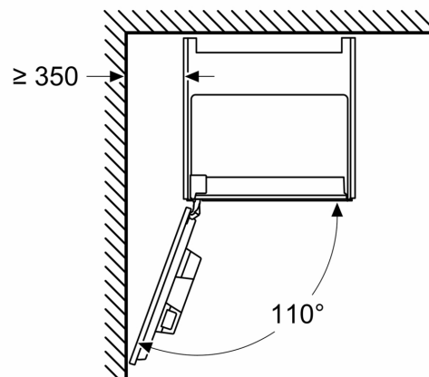
Maße in mm Eckeinbau links
