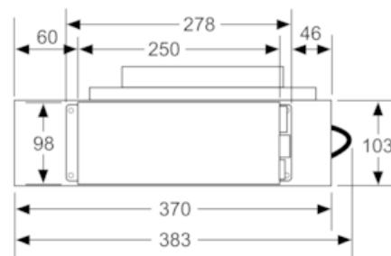
Ansicht Steuereinheit
