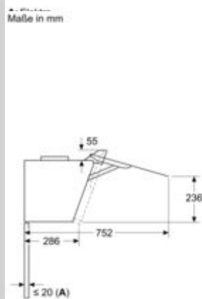
Maße in mm Gerät im Umluftbetrieb ohne Abluftkanal
