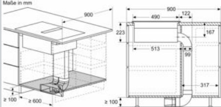
A: Adapterstück rund-flach
