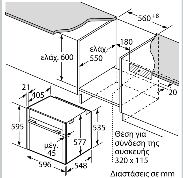
Διαστάσεις σε mm
