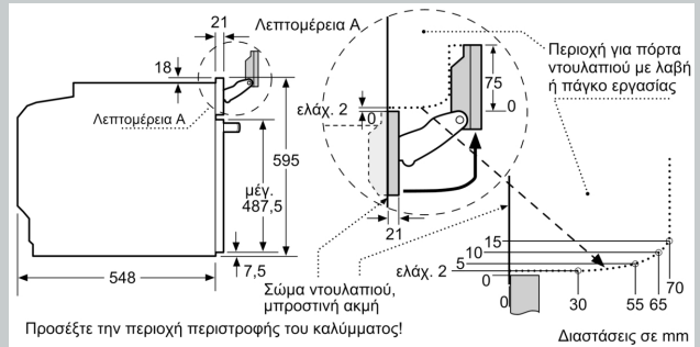
Διαστάσεις σε mm
