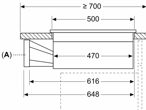
A: Προσαρμογέας στρογγυλός/επίπεδος
