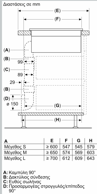
Διαστάσεις σε mm
