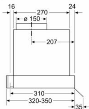
Dimensiones en mm Vista lateral
