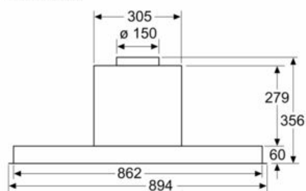
Dimensiones en mm Vista frontal
