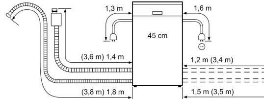
Medidas de conexión para todos los lavaplatos de 45 cm ( ) Valores con juego de prolongación Z 7710X0
