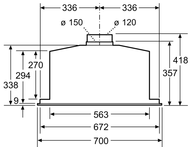
Mõõdud (mm)
