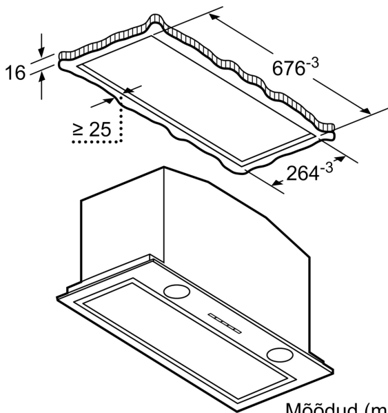
Mõõdud (mm)
