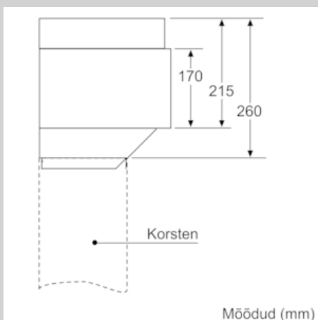
Mõõdud (mm)
