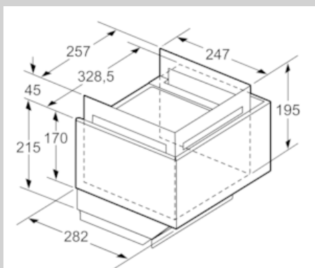
Mõõdud (mm)
