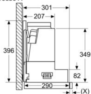
mjerne jedinice u mm Oblik izvedbe A
