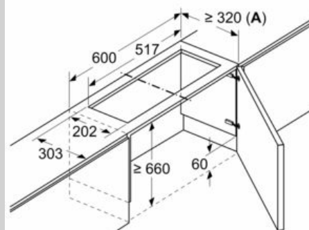
Mjere u mm Montaža teleskopske nape sa setom za kruženje zraka i okvirom za spuštanje
