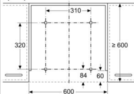
mjerne jedinice u mm
