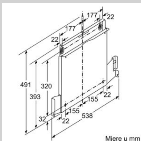
mjerne jedinice u mm
