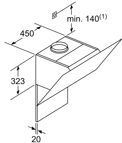
Méretetek mm-ben
