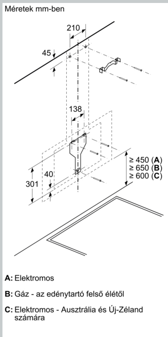
Méretetek mm-ben
