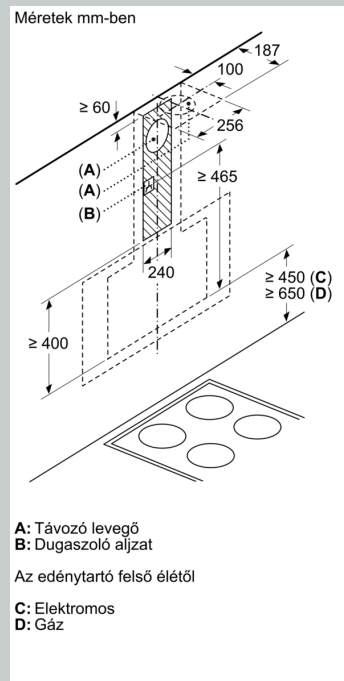
Méretetek mm-ben
