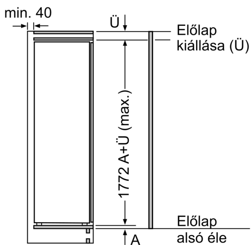
Méretetek mm-ben
