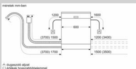
Méretetek mm-ben
