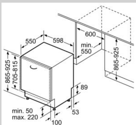
Méretetek mm-ben
