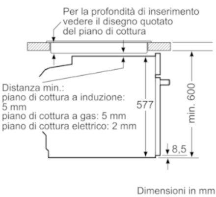
Montaggio con un piano di cottura.
