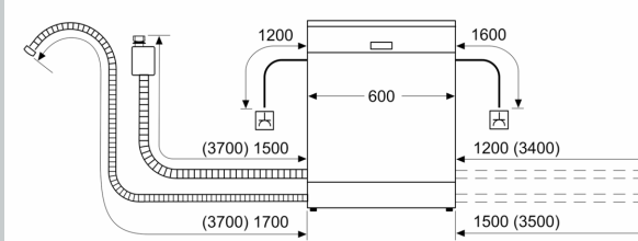
Dimensioni in mm
