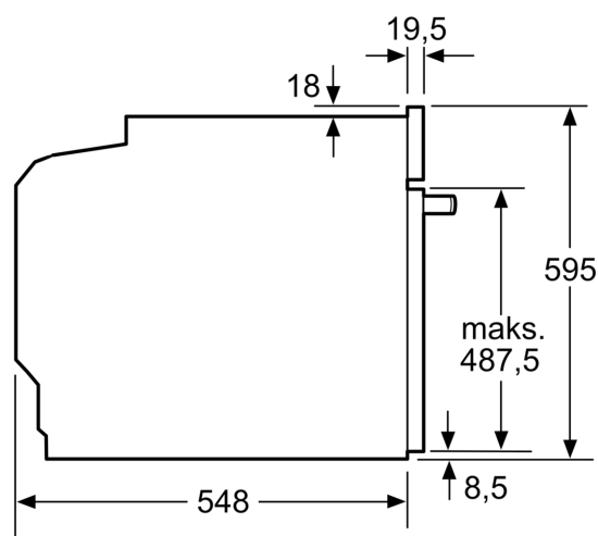
Matmenys, mm
