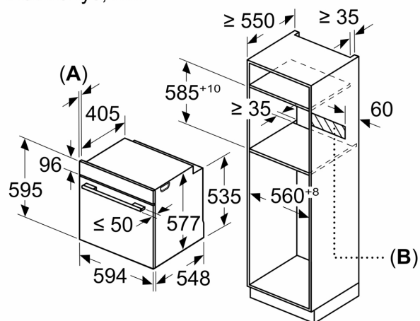
Matmenys, mm
