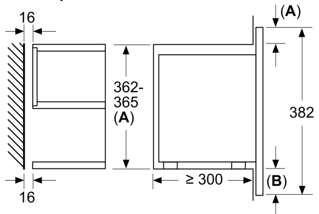
Matmenys, mm
