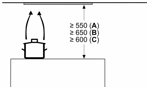
Matmenys, mm
