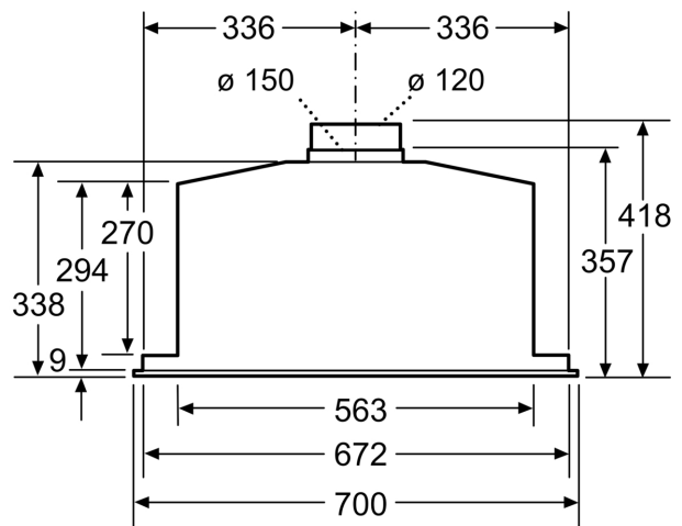
Matmenys, mm
