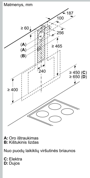
Matmenys, mm
