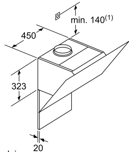
Matmenys, mm
