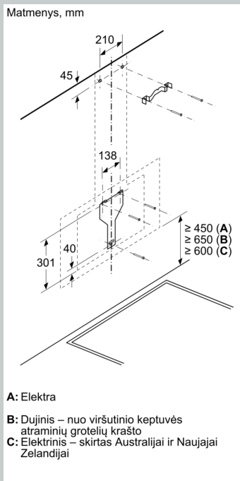
Matmenys, mm
