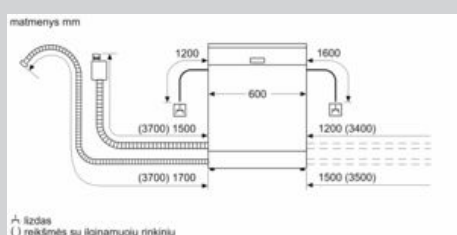
Matmenys, mm
