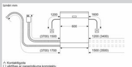
Izmēri (mm)
