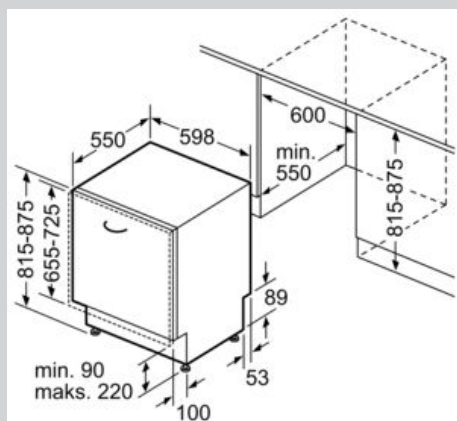
Izmēri (mm)
