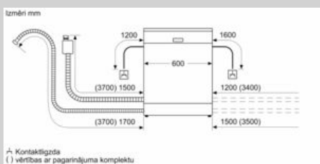
Izmēri (mm)
