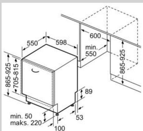
Izmēri (mm)
