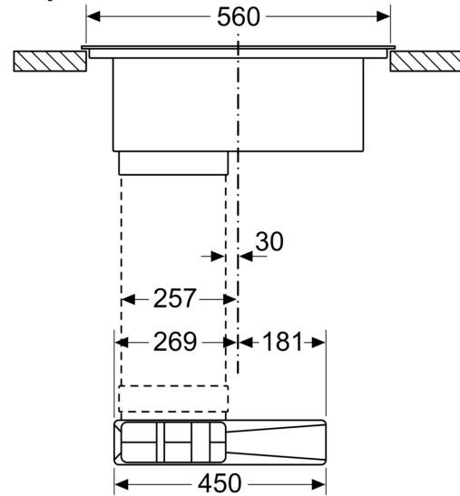
Izmēri (mm) Priekšējais skats
