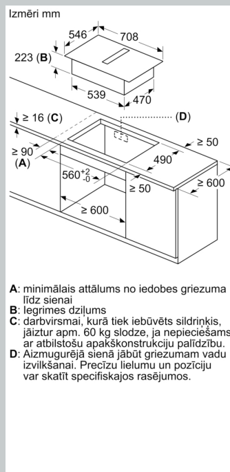
Izmēri mm Skats no priekšpuses - mēbeles izgriezums cirkulējošajam gaisam bez kanāla
