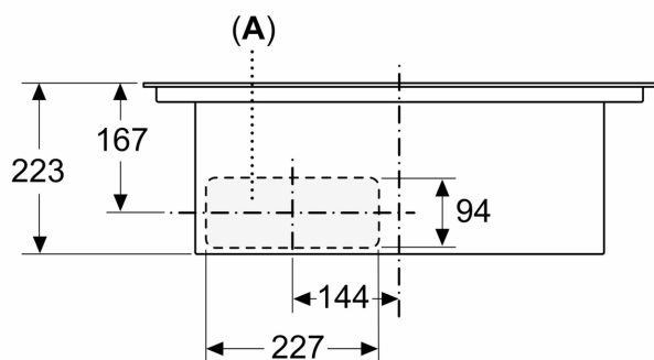
Izmēri mm Skats no priekšpuses
