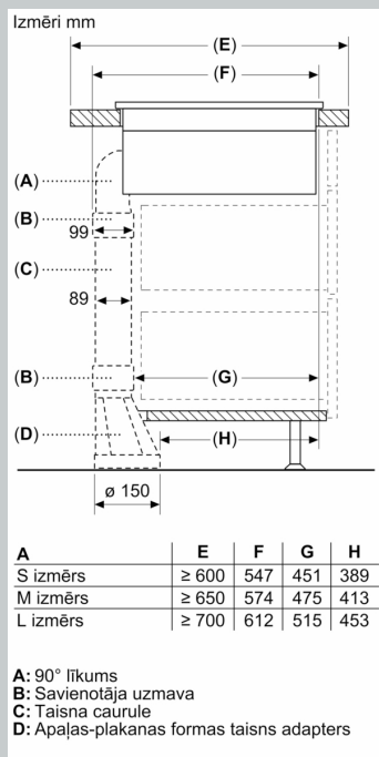
Izmēri mm Skats no priekšpuses
