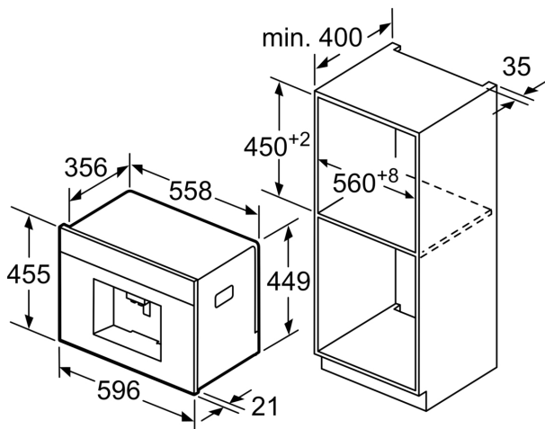
Bønne- og vannbeholderne tas ut forfra. Anbefalt innbyggingshøyde 95-145 cm.
