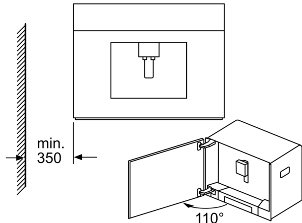
Ved bruk av 92° hengsel- stopper (reservedelsnr. 00636455) er minsteavstanden til veggen bare 100 mm.
