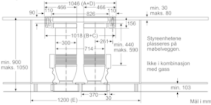
Kombinasjon 2*vifteelement 1*platetopp 80 cm
