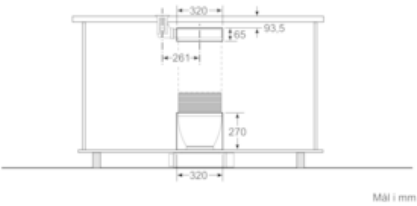
Utskjæring i bakstykke
