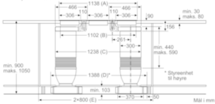
Kombinasjon 2*vifteelement 3*domino-enheter 30 cm
