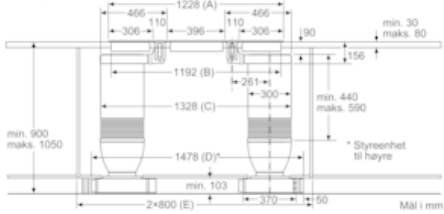
Kombinasjon 2*vifteelement 2*domino-enheter 30 cm 1*domino-enhet 40 cm
