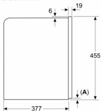
Dimensiuni în mm
