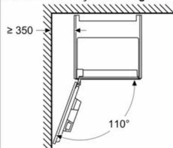
Dimensiuni în mm
