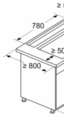
Mått i mm Kombination med Förhöjd standardr
