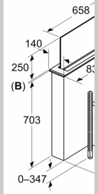
Mått i mm
